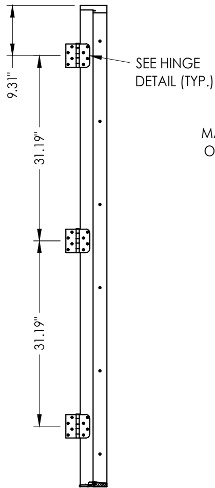
STRIKE JAMB
